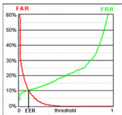
Рис. 1. Связь между FRR и FAR
