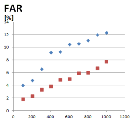
Рис. 3. FAR емкостного дактилоскопического датчика
