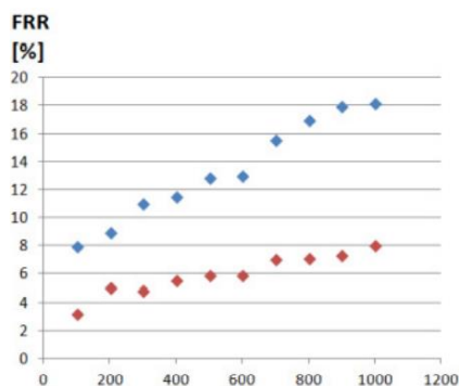
Рис. 2. FRR емкостного дактилоскопического датчика
